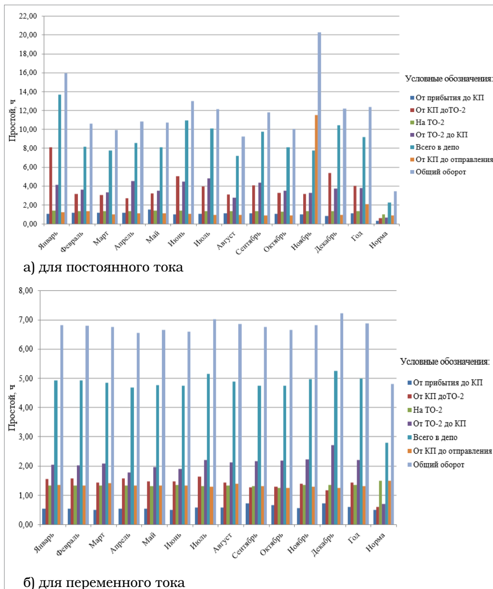
Рис. 2. Динамика фактических значений времени оборота поездных локомотивов
