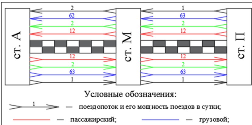
Рис. 1. Диаграмма расчетных среднесуточных поездопотоков на основе существующих размеров движения Восточного полигона железных дорог
